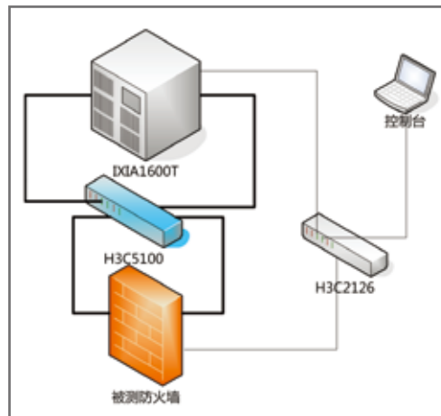
图3. 测试仪器配置方案2
