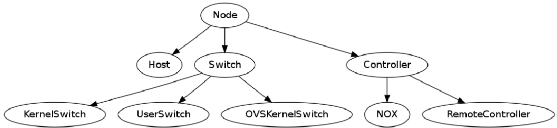
图表 5-3 node.py 类继承关系
