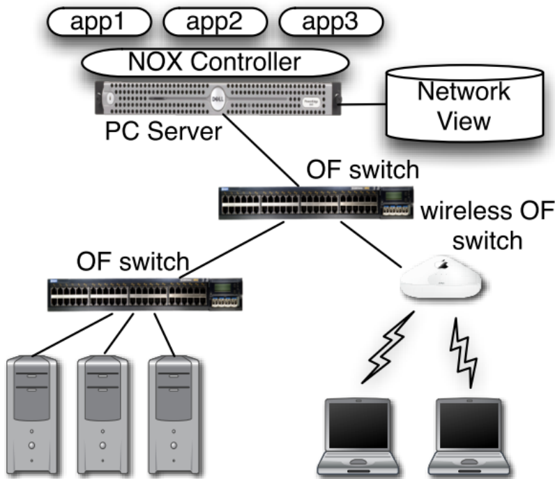
图表 4-1 NOX 管理网络的主要部件
