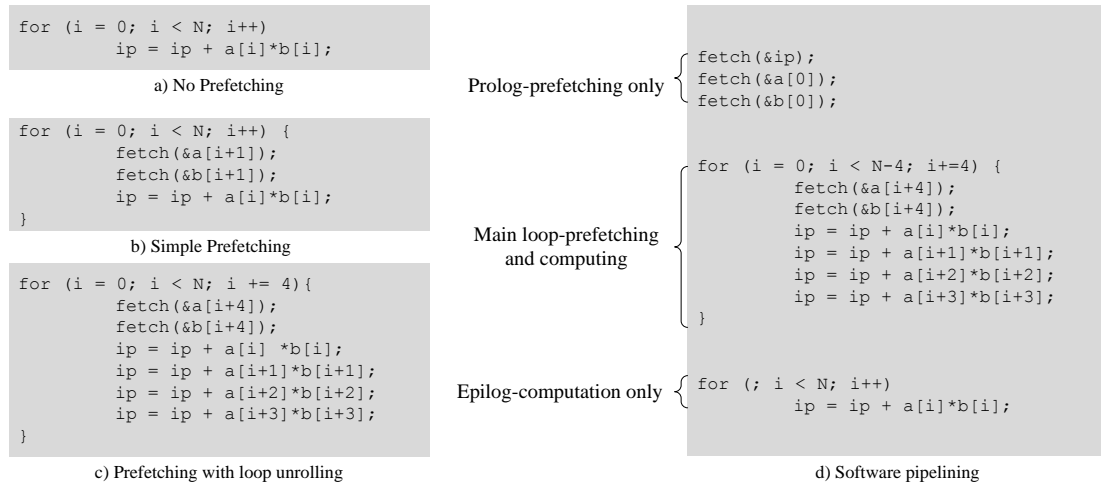
图 5-2 利用软件预读指令进行程序优化[100]
