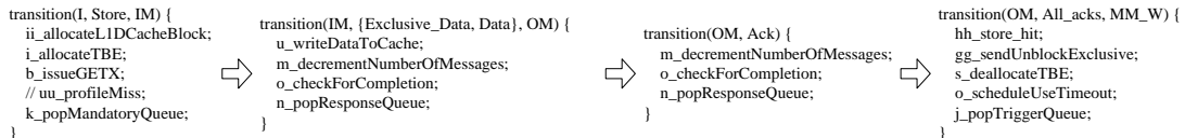
图 4-14 状态 I 至 MM_W 的迁移过程
