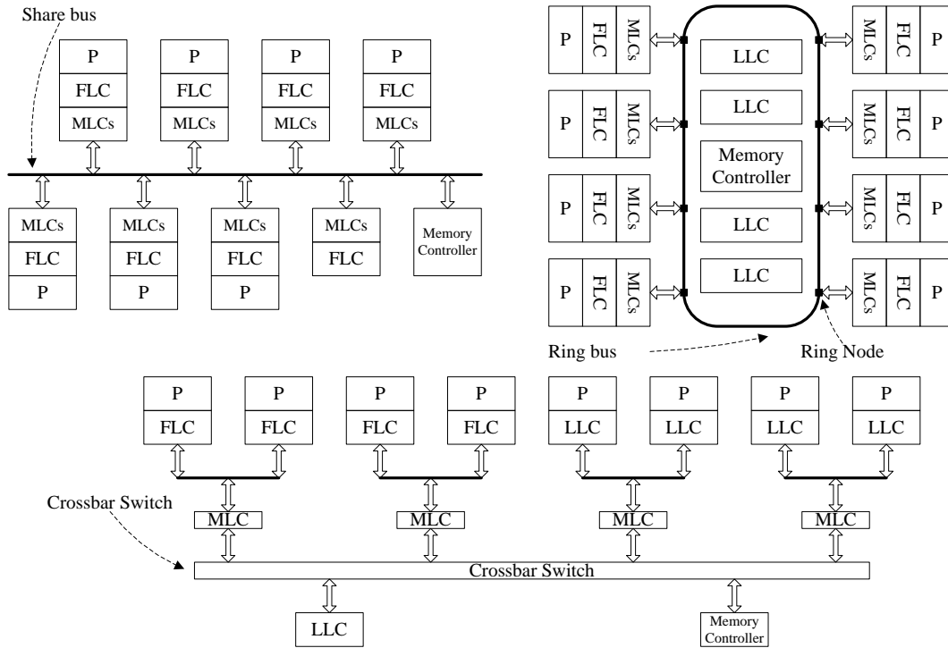
图 4-5 CPU Core 与 Cache Hierarchy 的连接通路
