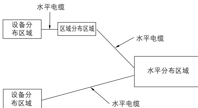
图7 典型的星状布局水平电缆
