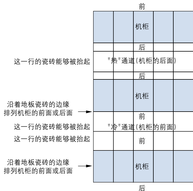
图6 “热”通道,“冷”通道和机柜放置范例
