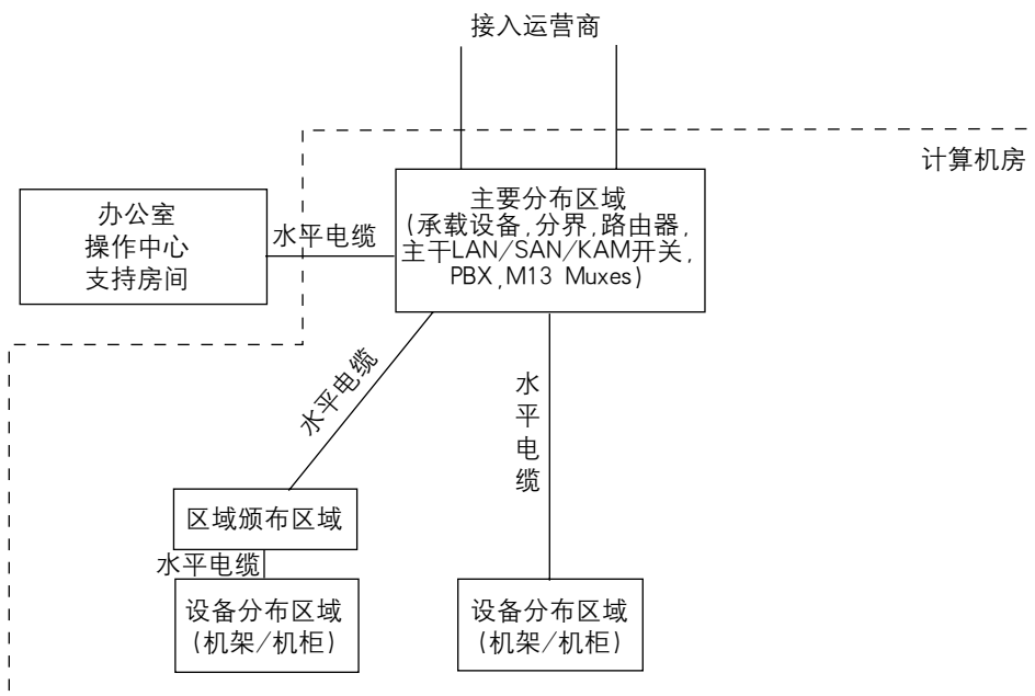
图4 简化的数据中心布局范例
