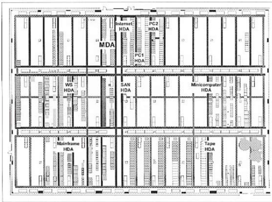
(图 21: 公司数据中心范例)
