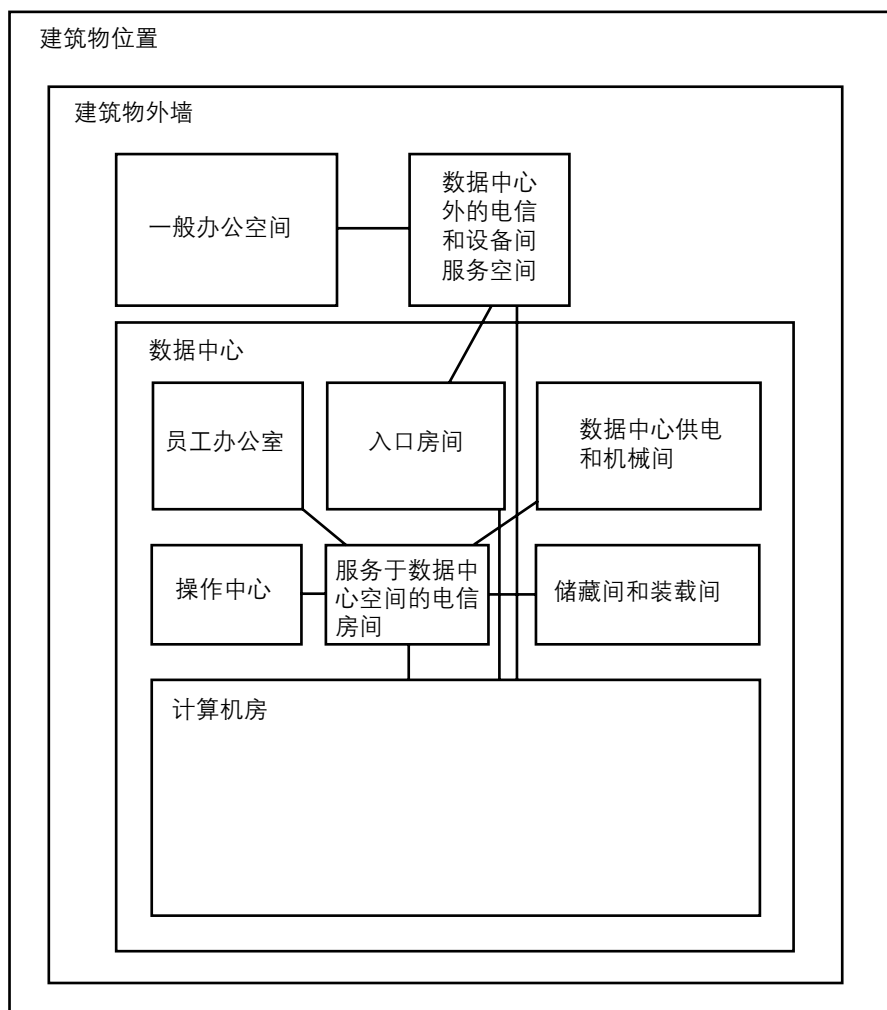
图1 数据中心的空间关系
