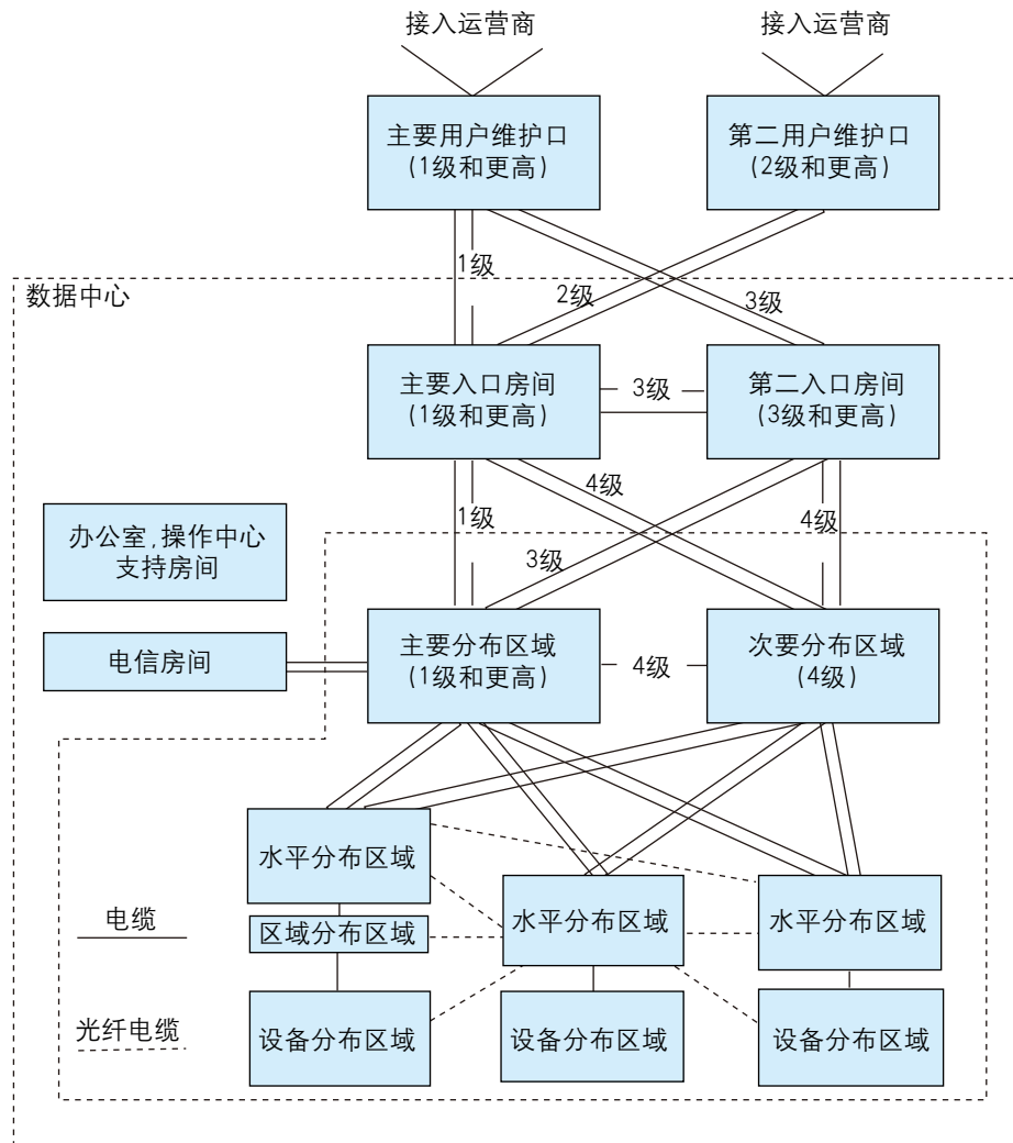
图10 电信基础设施冗余
