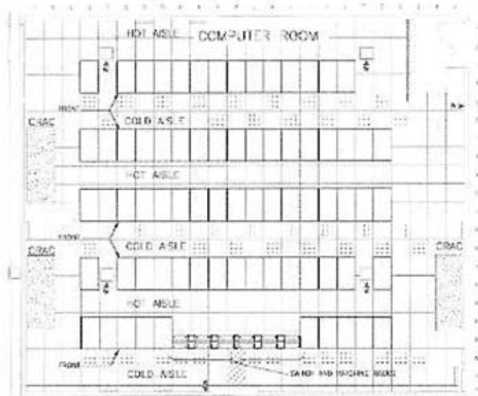
(图20: 显示“热”和“冷”通道的计算机房规划图)
