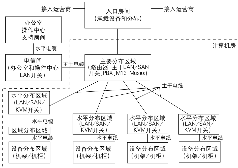
图3 基本的数据中心布局范例
